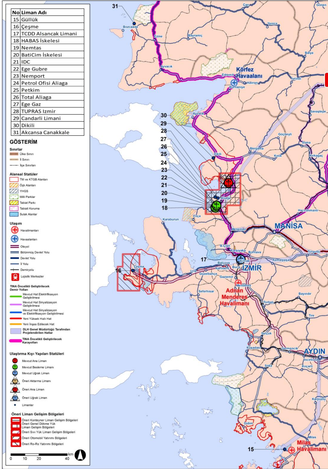
Şekil B.7.3. Ege Bölgesi Öneri Liman Gelişim Bölgeleri
