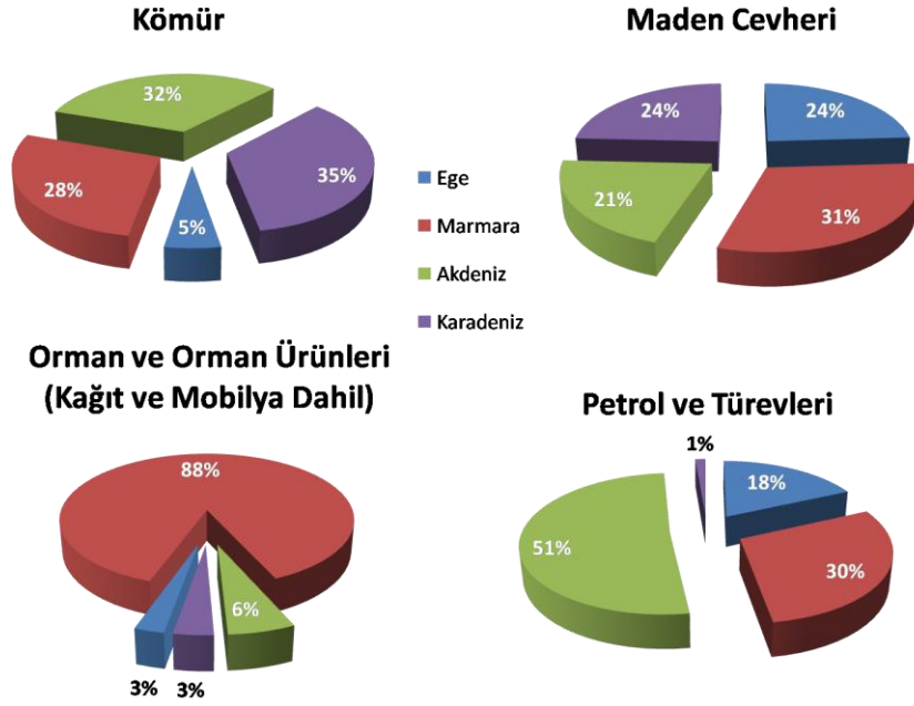
Grafik B.3.32: Limanlarımızda Elleçlenen Yüklerin Bölgelere Göre Dağılımı (Kömür, maden cevheri, orman ve orman ürünleri, petrol ve türevleri)
