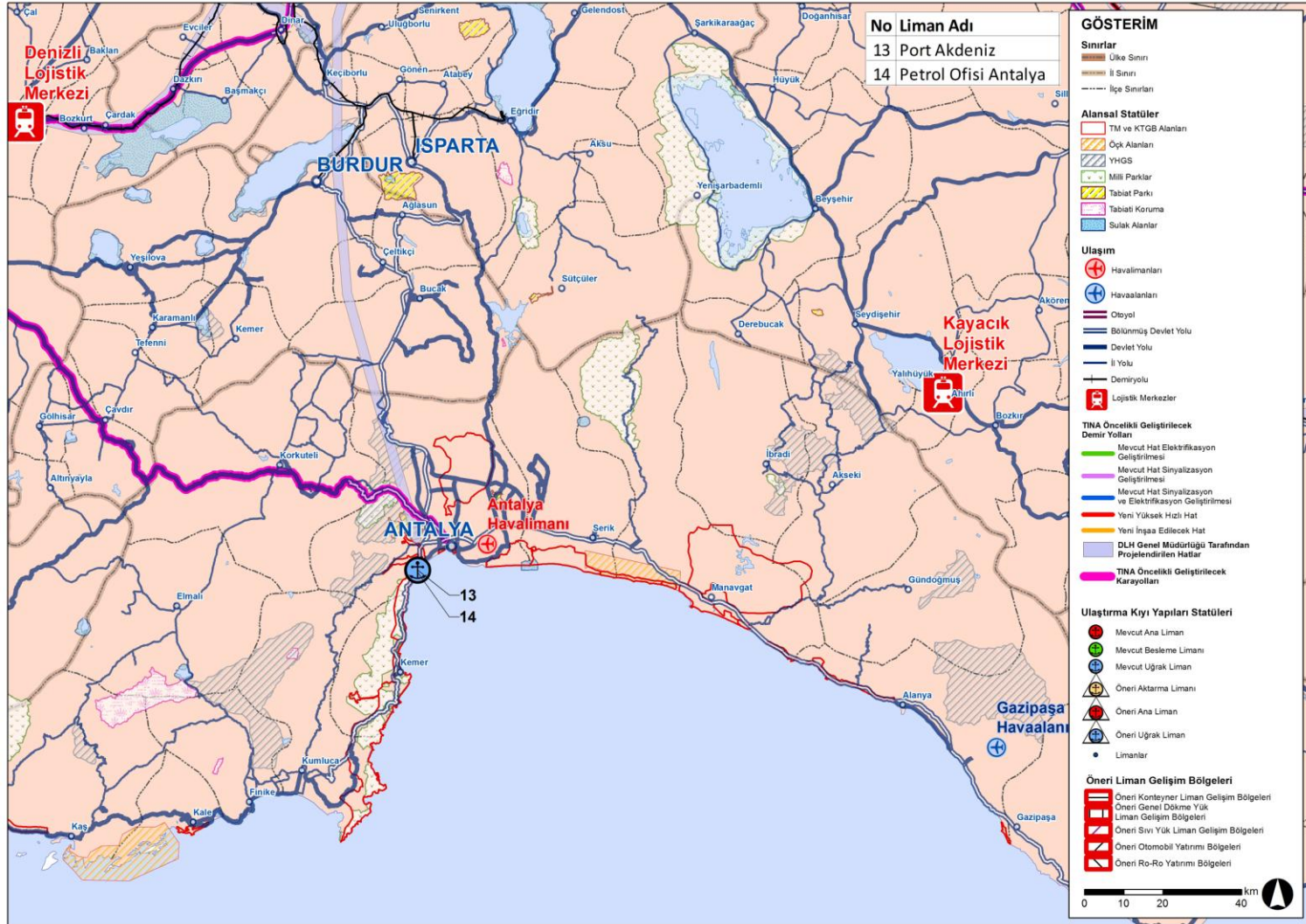
Şekil B.7.2. Doğu Akdeniz Bölgesi Öneri Liman Gelişim Bölgeleri
