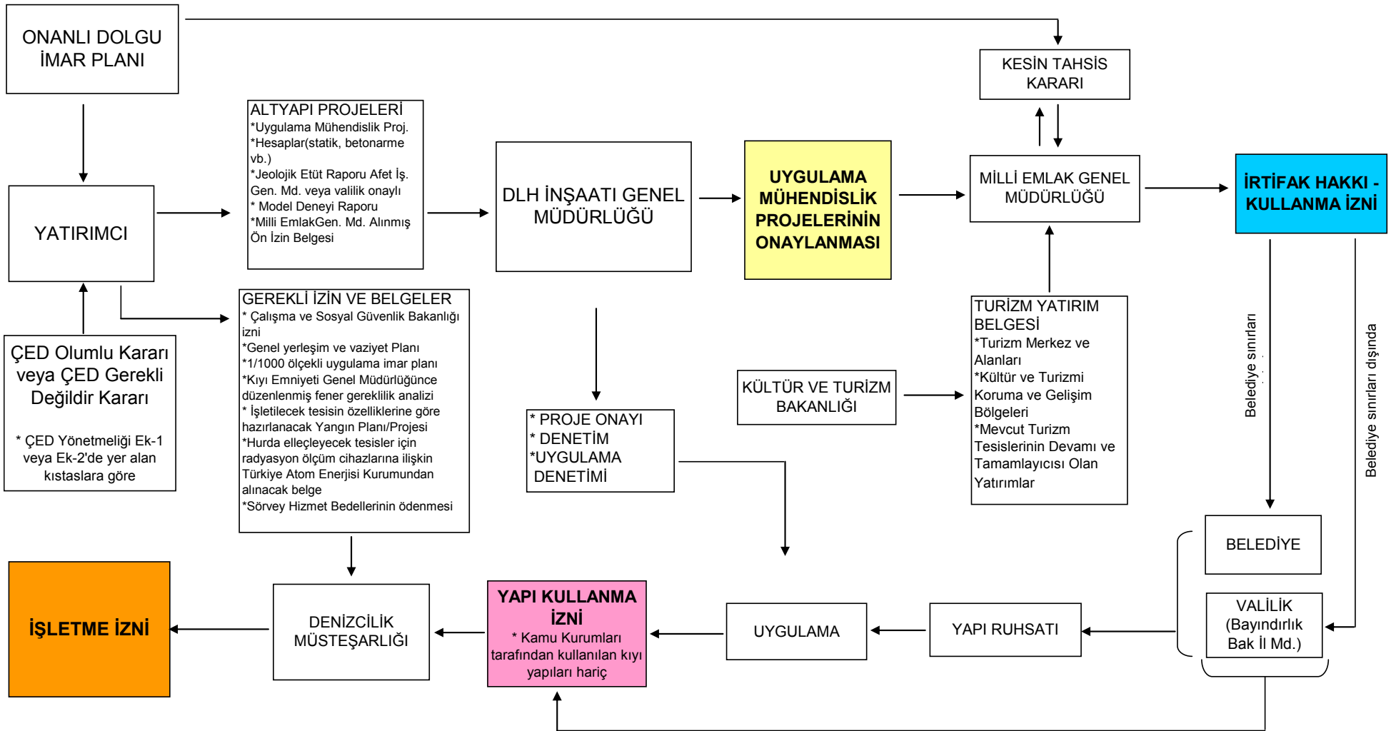
Şekil B.6.2. Kıyı Yapıları Proje ve Uygulama Süreci
