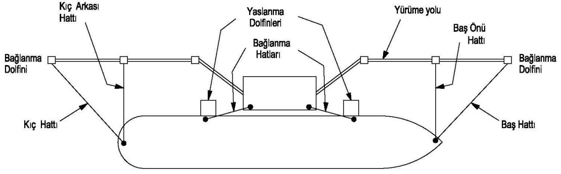
Şekil EK 1.4: T tipi iskelede bağlanma
