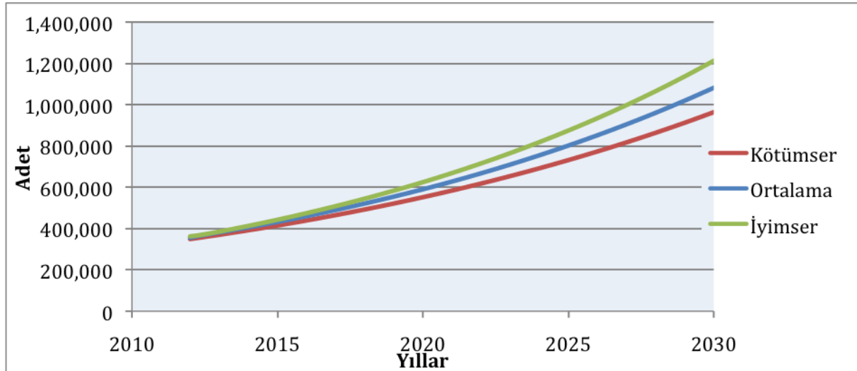
Grafik B.3.22: Harici Ro-Ro Yük Elleçlemesinin 2015-2030 Tahmini Grafiği (Adet)
