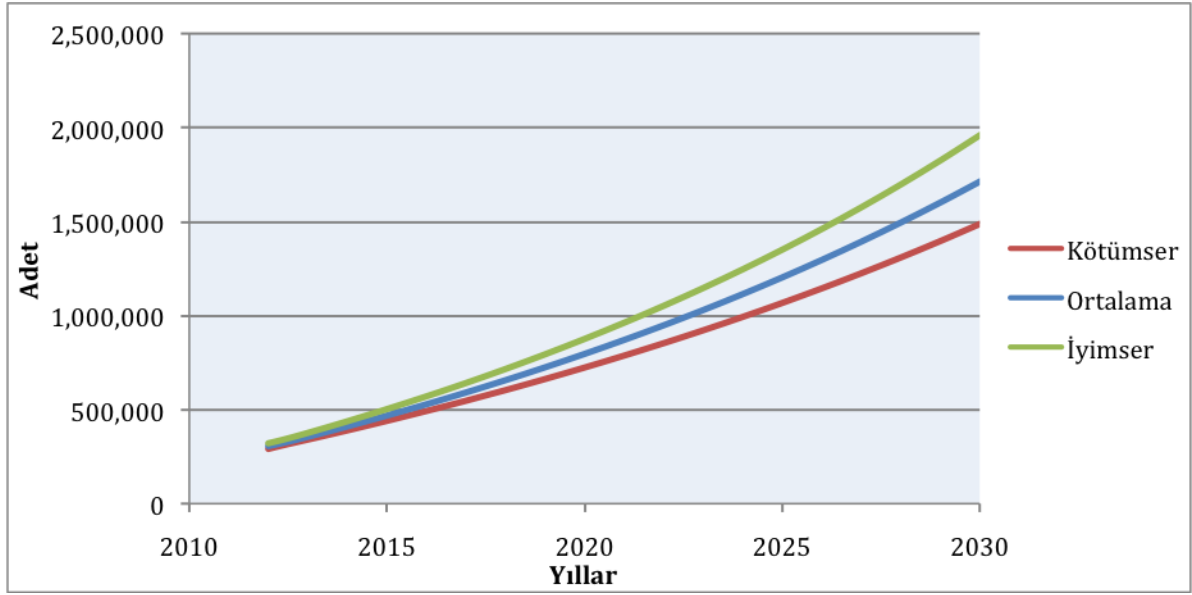
Grafik B.3.29: Marmara Bölgesinde Elleçlenecek Dahili Ro-Ro Yükünün Tahmini (Adet)
