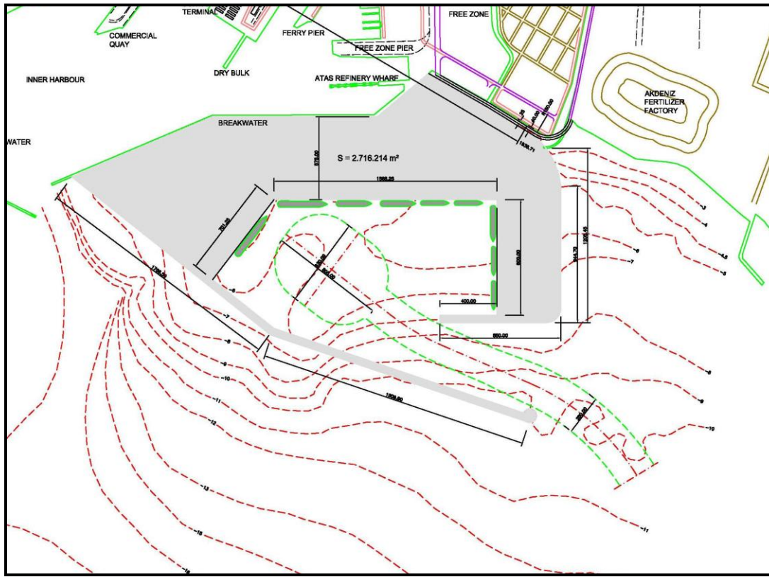
Şekil EK 4.2: Mersin Limanı Fizibilite Çalışması Önerilen Yeni Liman Yerleşimi
