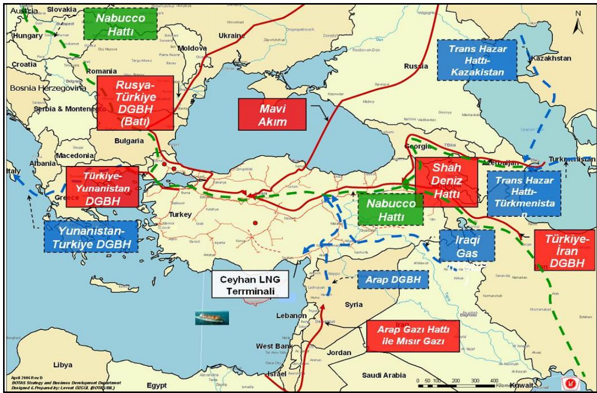
Şekil A.2.7: Uluslararası Doğal Gaz Boru Hattı Projeleri
