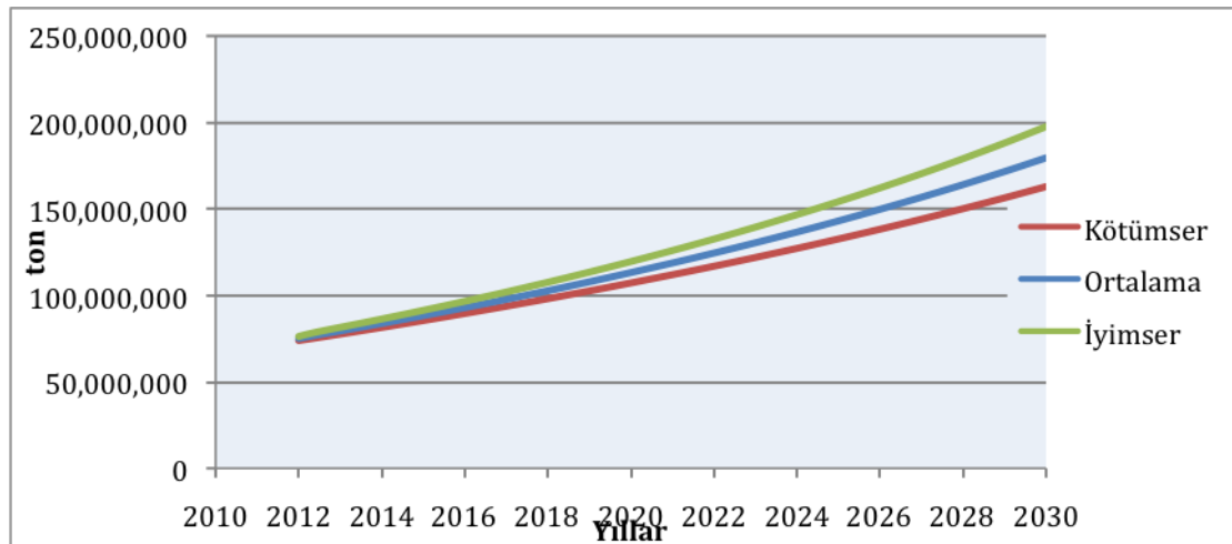
Grafik B.3.17: Sıvı Dökme Yük Elleçleyen Türkiye Limanlarının 2015-2030 Yıllarına Ait Toplam Yük Tahmini Grafiği
