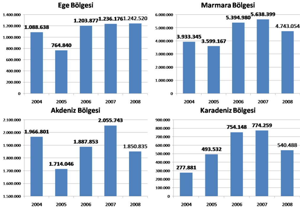
Grafik B.3.45: Türkiye Limanlarında Elleçlenen Endüstriyel Ürünler ve Ham Maddelerin Bölgelere Göre Yıllık Değişimi (2004 – 2008)
