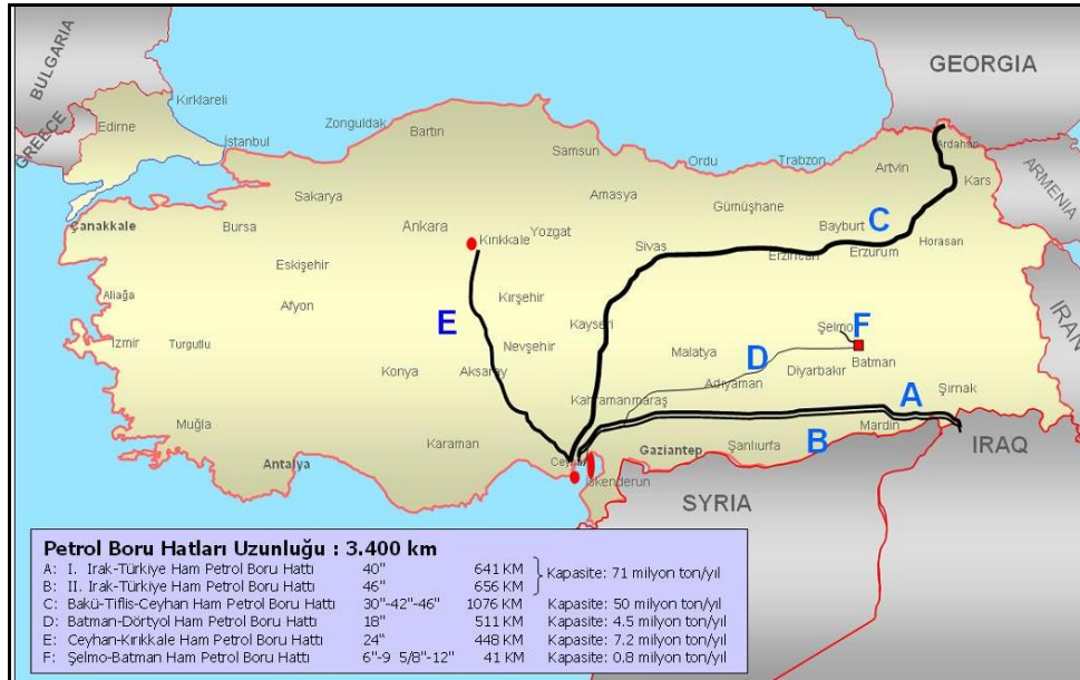
Şekil A.2.5: Türkiye'de Ham Petrol Boru Hatları
