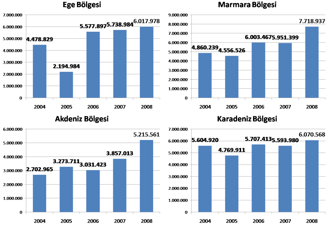
Grafik B.3.41: Türkiye Limanlarında Elleçlenen Maden Cevherinin Bölgelere Göre Yıllık Değişimi (2004 – 2008)
