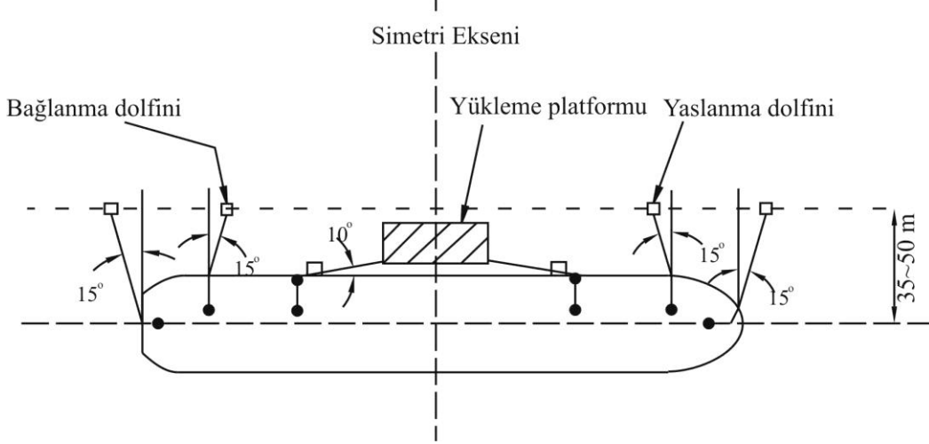
Şekil EK 1.5: Yükleme platformuna bağlanan tankerin bağlanma düzeni
