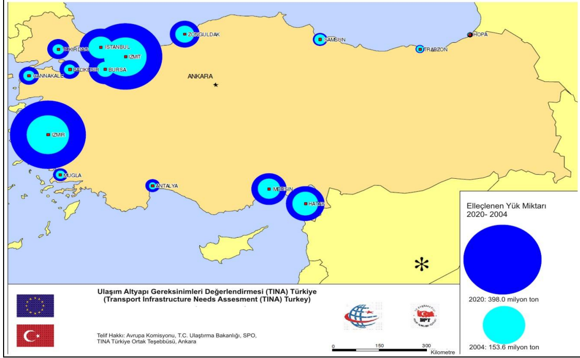
Şekil EK 5.18: Ana Limanlar Elleçleme Miktarları, Referans Senaryo 2020,
