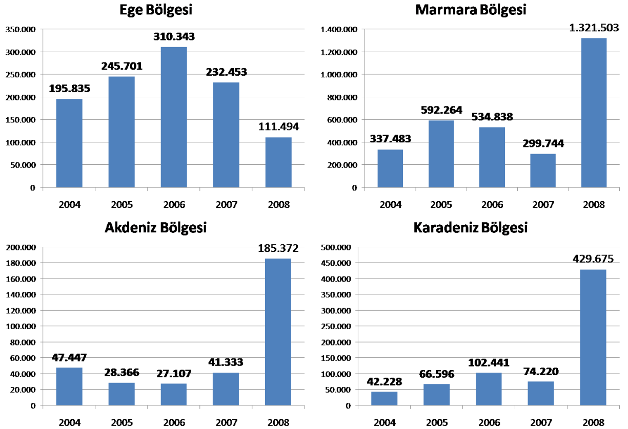
Grafik B.3.49: Türkiye Limanlarında Elleçlenen İnşaat ve Yapı Malzemelerinin Bölgelere Göre Yıllık Değişimi (2004 – 2008)
