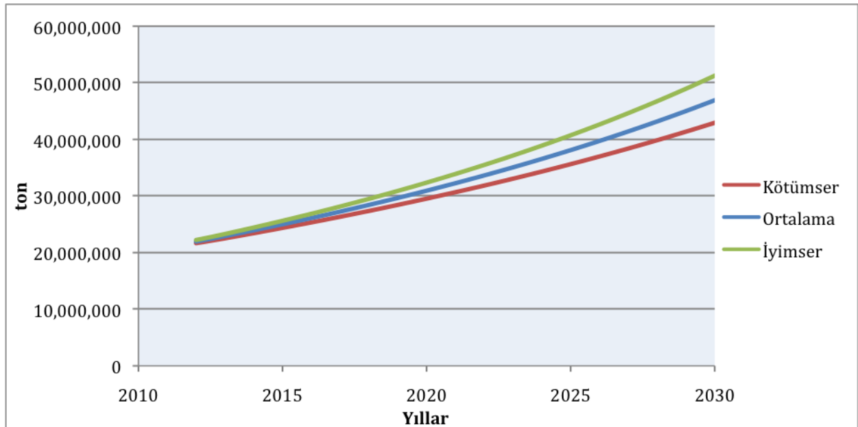
Grafik B.3.19: Ege Bölgesinde 2015-2030 Yılları Arasında Elleçlenecek Sıvı Yükün Tahmini Grafiği (Ton)
