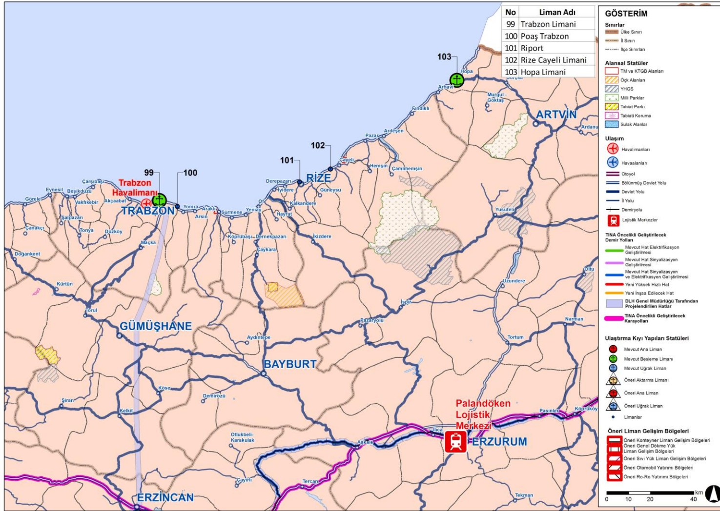
Şekil B.7.7. Doğu Karadeniz Bölgesi Öneri Liman Gelişim Bölgeleri
