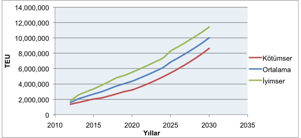
Grafik B.3.10: Akdeniz Bölgesinde 2015-2030 Yılları Arasında Elleçlenecek, Aktarma Dahil, Toplam Konteynerin Tahmini Grafiği (TEU)
