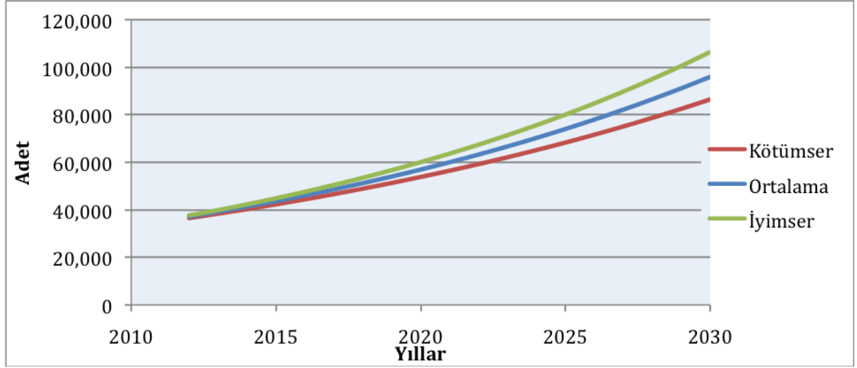
Grafik B.3.26: Ege Bölgesi'nde Elleçlenecek Harici Ro-Ro Yükünün Tahmini Grafiği (Adet)
