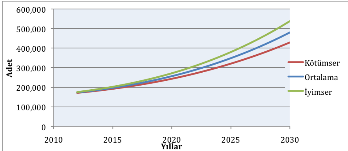
Grafik B.3.25: Marmara Bölgesinde Elleçlenecek Harici Ro-Ro Yükünün Tahmini
