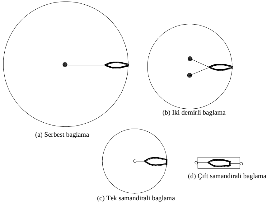
Şekil EK 1.3: Her bir gemi için şamandıralara bağlanma alanı için temel tasarım
