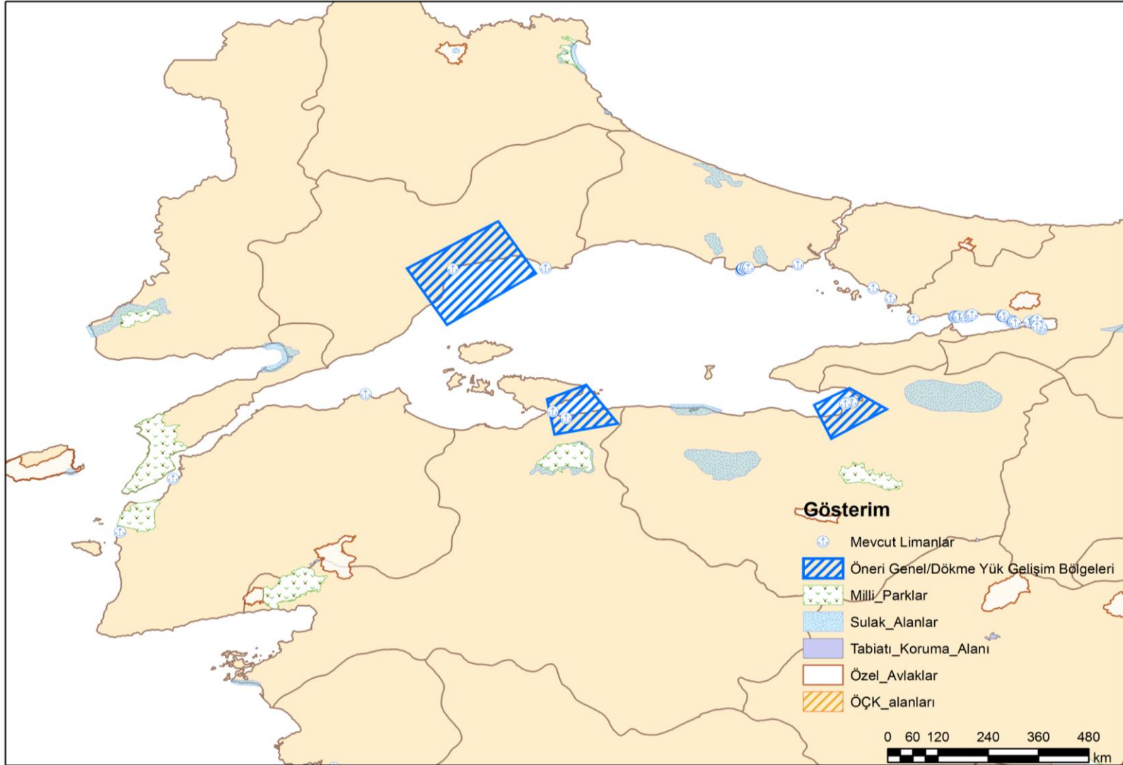
Şekil B.5.6: Marmara Bölgesi Genel/Dökme Yük Limanları ve Yeni Yatırımlar için Öneriler
