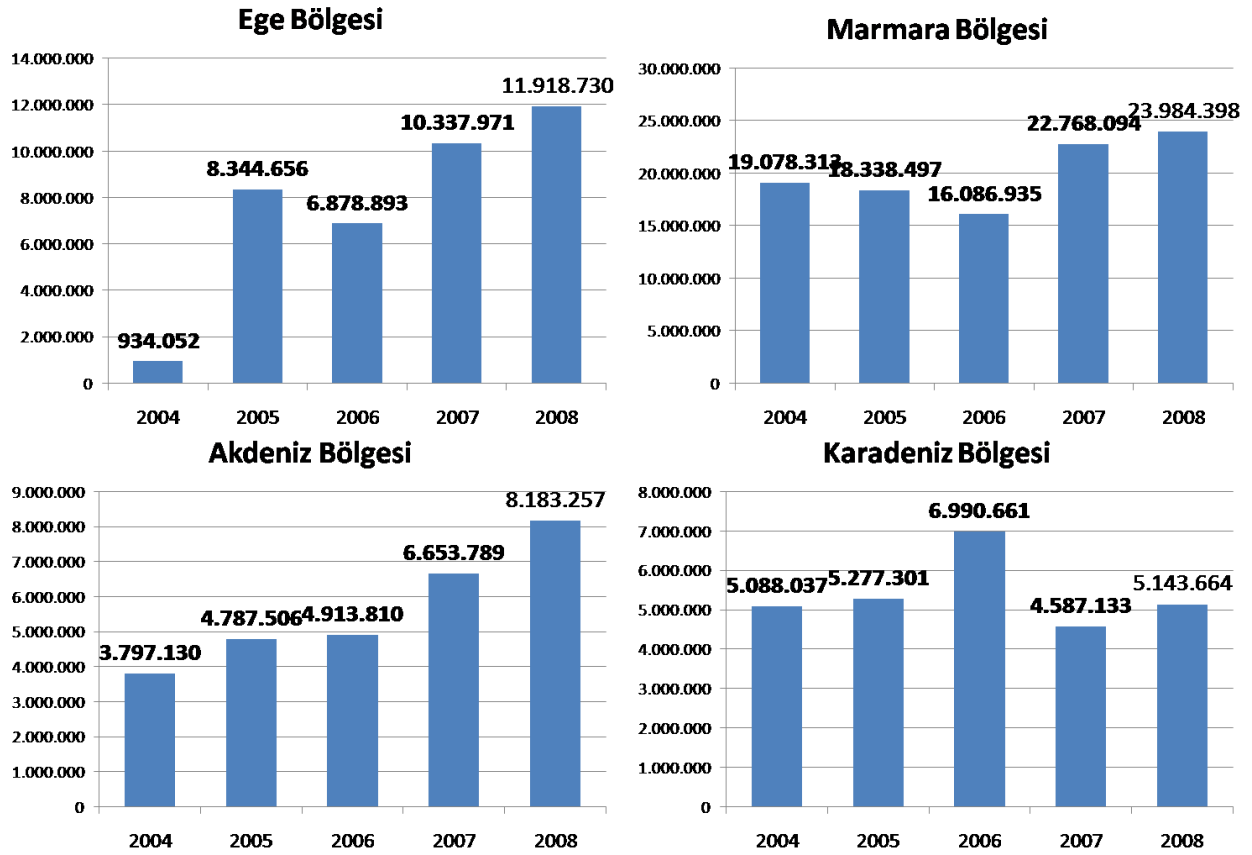
Grafik B.3.40: Türkiye Limanlarında Elleçlenen Demir Çelik Ürünlerinin Bölgelere Göre Yıllık Değişimi (2004 – 2008)
