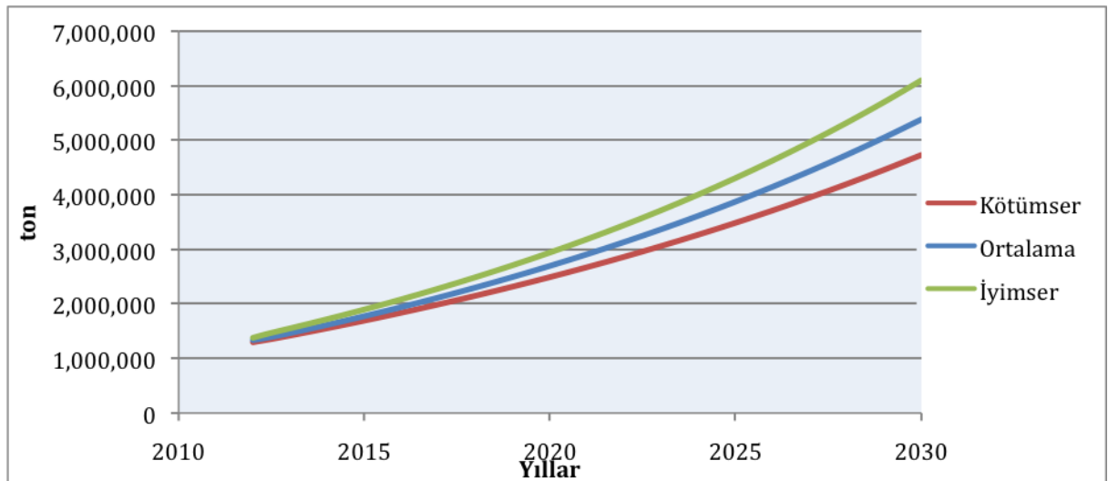
Grafik B.3.21: Karadeniz Bölgesinde 2015-2030 Yılları Arasında Elleçlenecek Sıvı Yükün Tahmini Grafiği (Ton)
