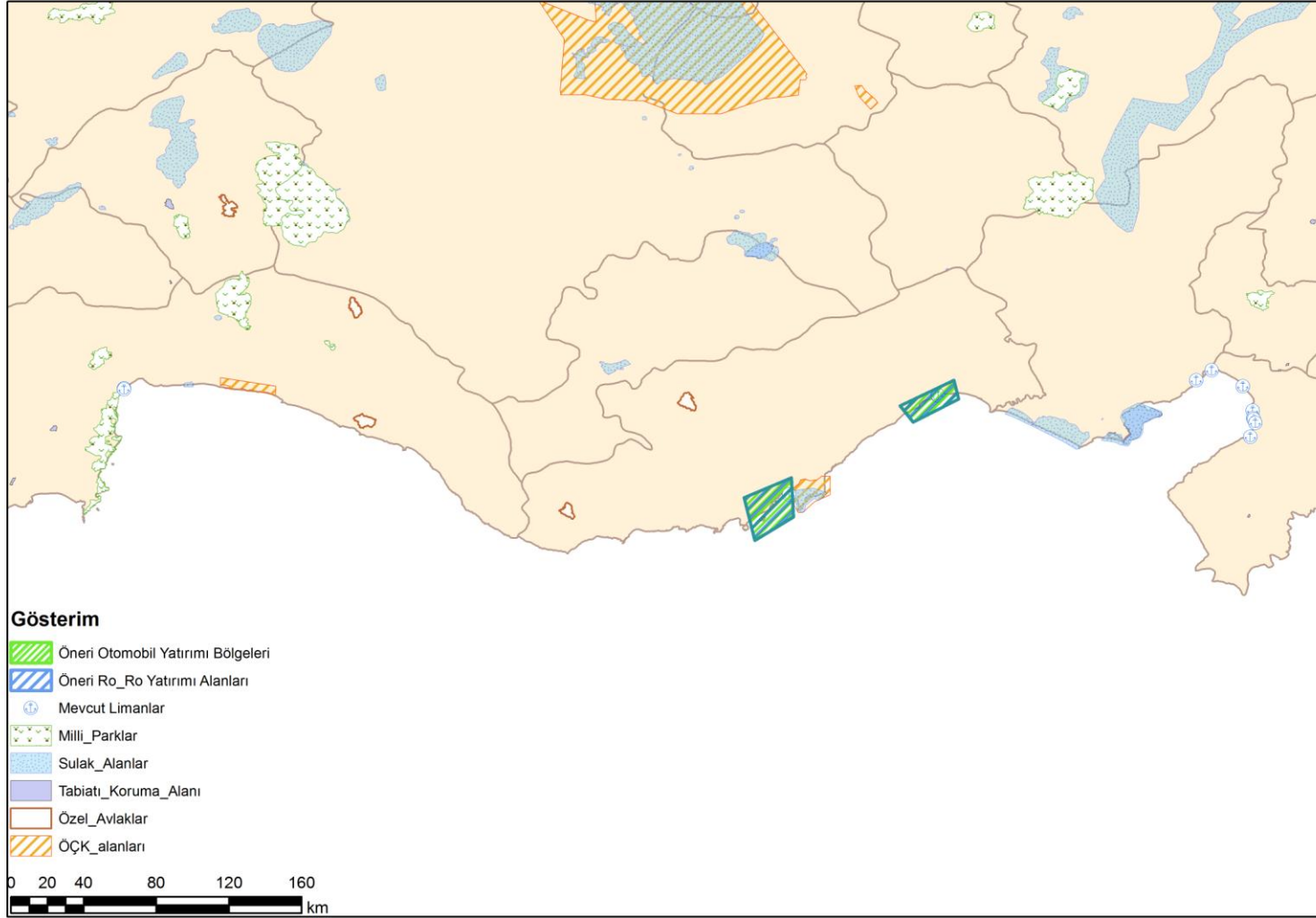
Şekil B.5.13: Akdeniz Bölgesi Otomobil ve Ro-Ro Elleçlemesi için Yeni Yatırım Bölgesi Önerileri
