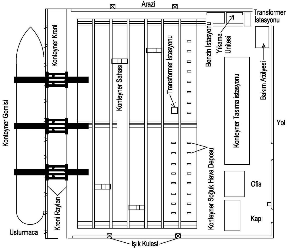
Şekil EK 1.1:Tipik Konteyner Terminali İşletme Planı
